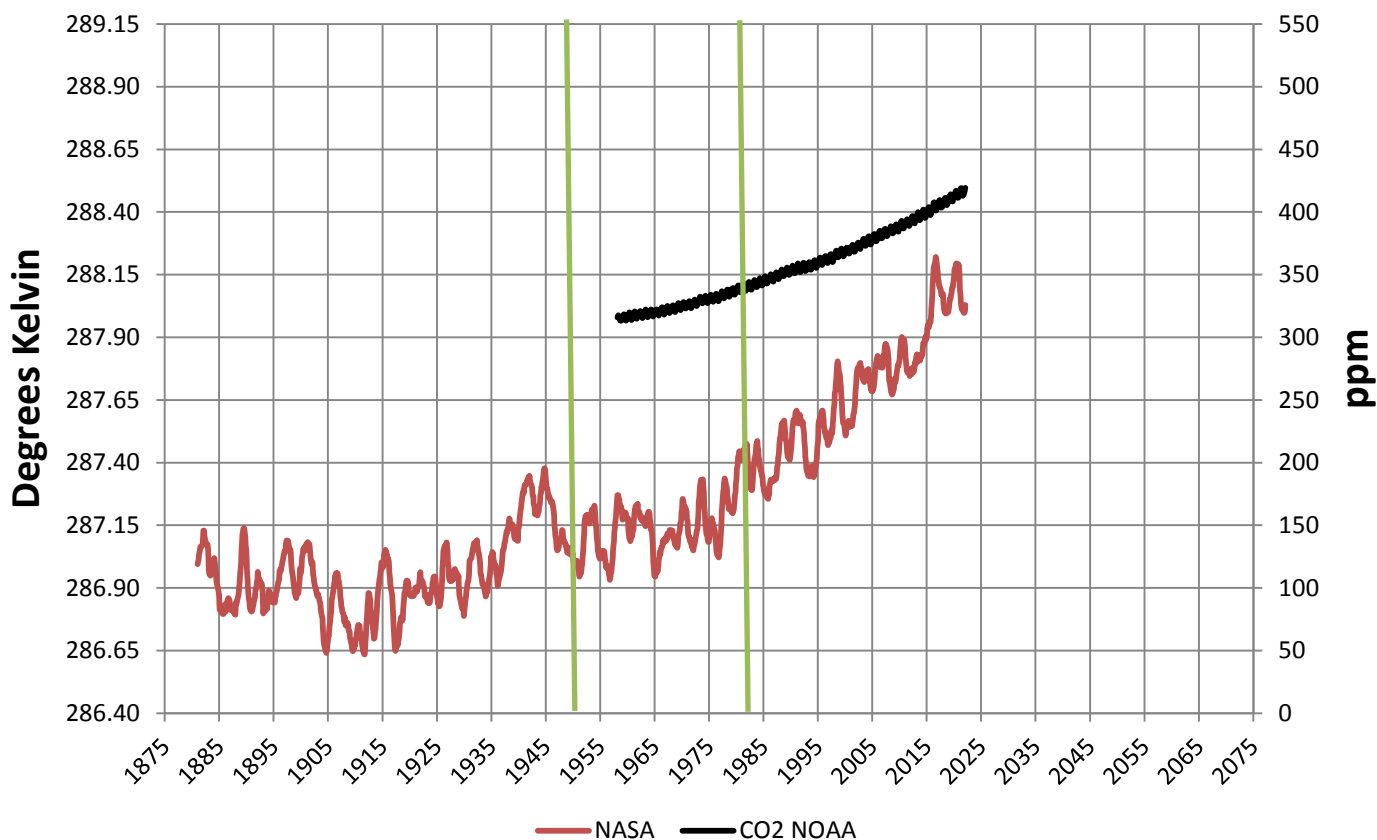
Chart 1b, NASA and NOAA actual numbers
