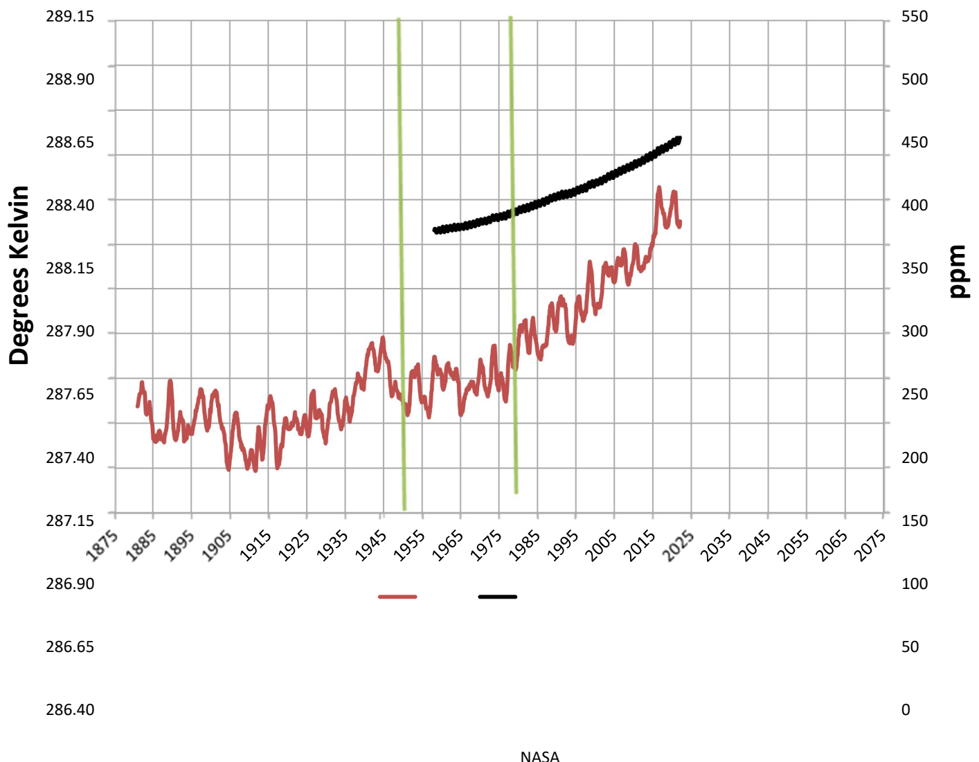
Chart 1b, NASA and NOAA actual numbers
